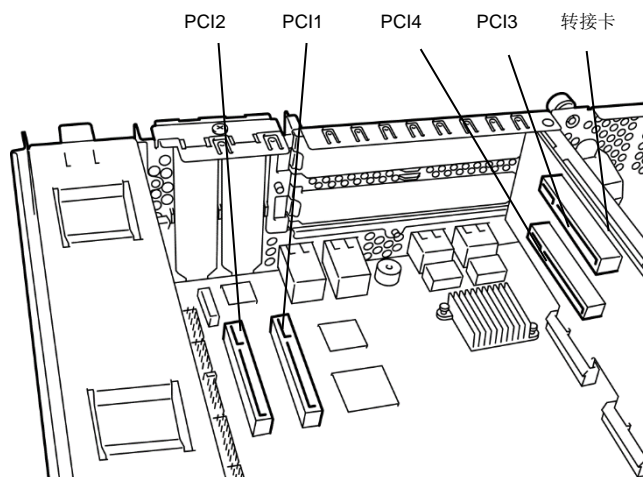
< R320e-M4 型号, R320f-M4 (附带转接卡) >
