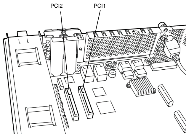
R320g-E4 型号 (不带 PCI 转接卡)
