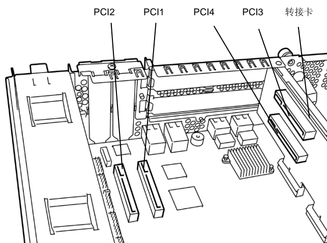
R320g-M4 型号 (带 PCI 转接卡)
