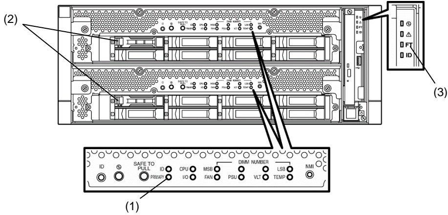
[CPU 模块重复时的状态指示灯的显示]
