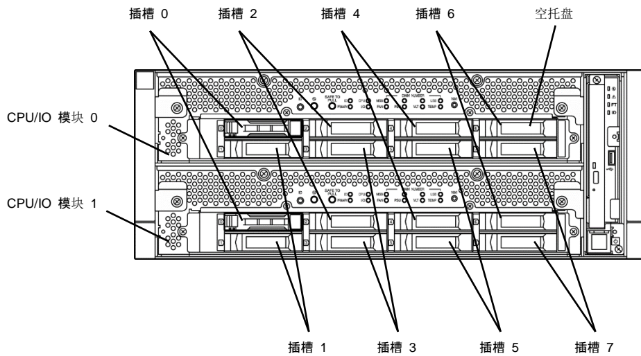
与镜像过程相关的插槽
