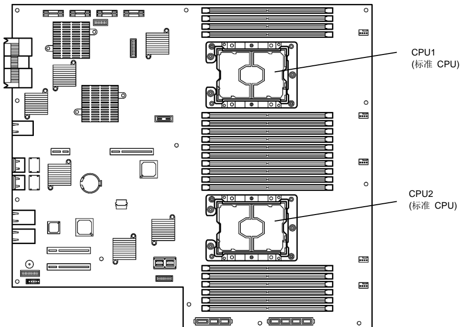
CPU / IO 模块中的 CPU 插槽
