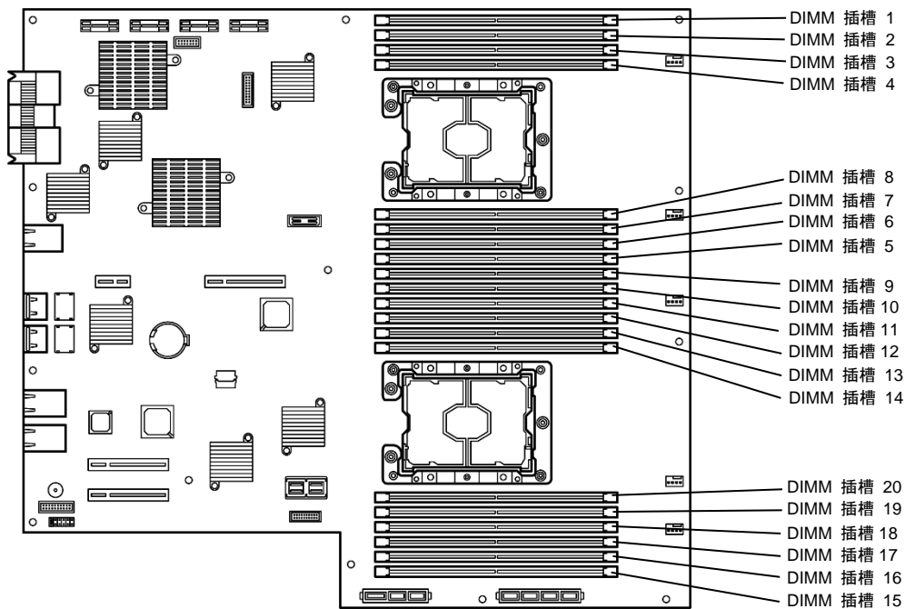
CPU/IO 模块中的 DIMM 插槽
