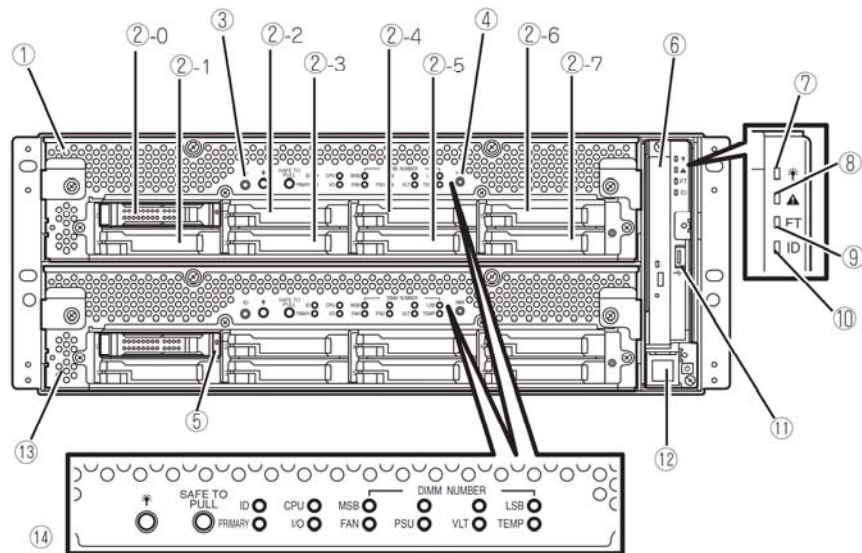
拆下前面板
