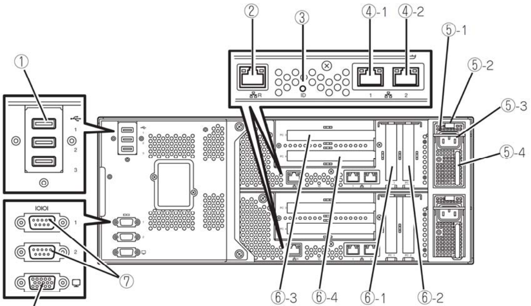
R320b-M4
