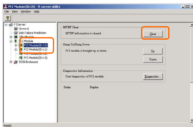
[PCI Module]
