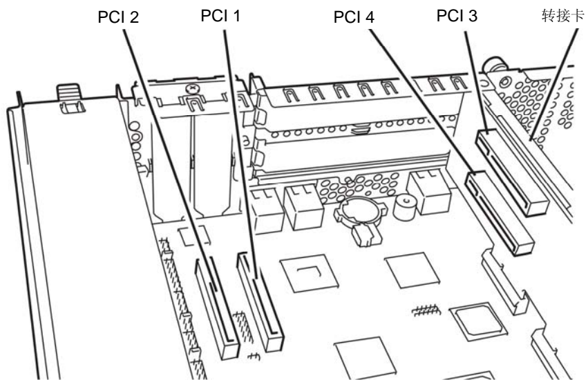
R320b-M4
